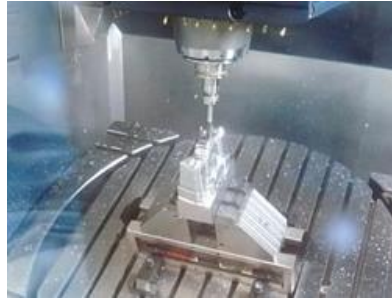
中型5軸加工機
